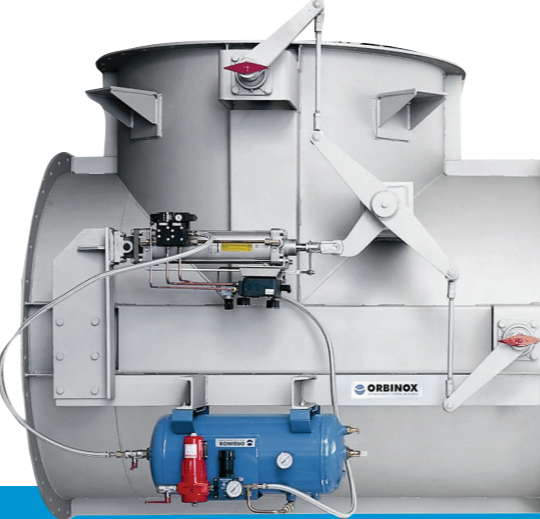
DI Multiple diverter damper
